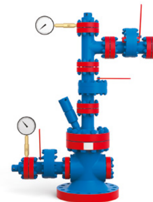
АФК1(Ш)-65x21К1(К2)М4-05 Без лубрикаторной задвижки и задвижки на боковом отводе крестовины
