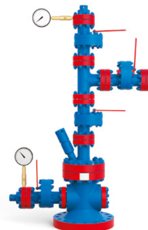
АФК1(Ш)-65x21К1(К2)М4-03 Без задвижки на боковом отводе крестовины
