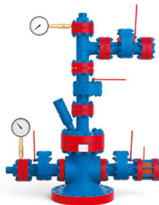
АФК1(Ш)-65x21К1(К2)М4-01 Без лубрикаторной задвижки
