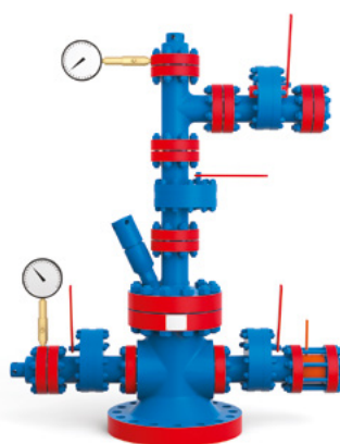
АФК1(Ш)-65x21K1(K2)M4-01 Без лубрикаторной задвижки
